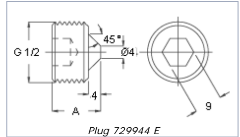
Plug 729944 E
