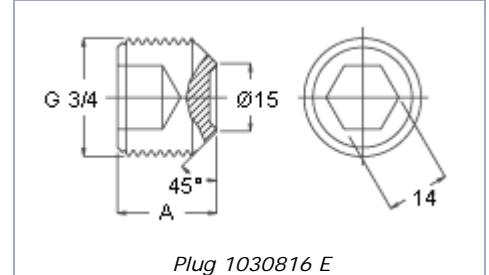
Plug 1030816 E
