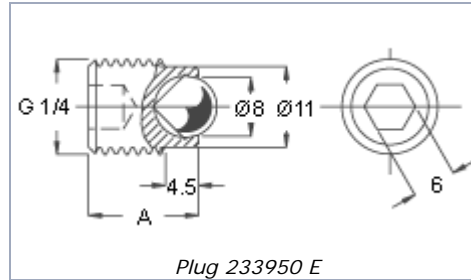
Plug 233950 E
